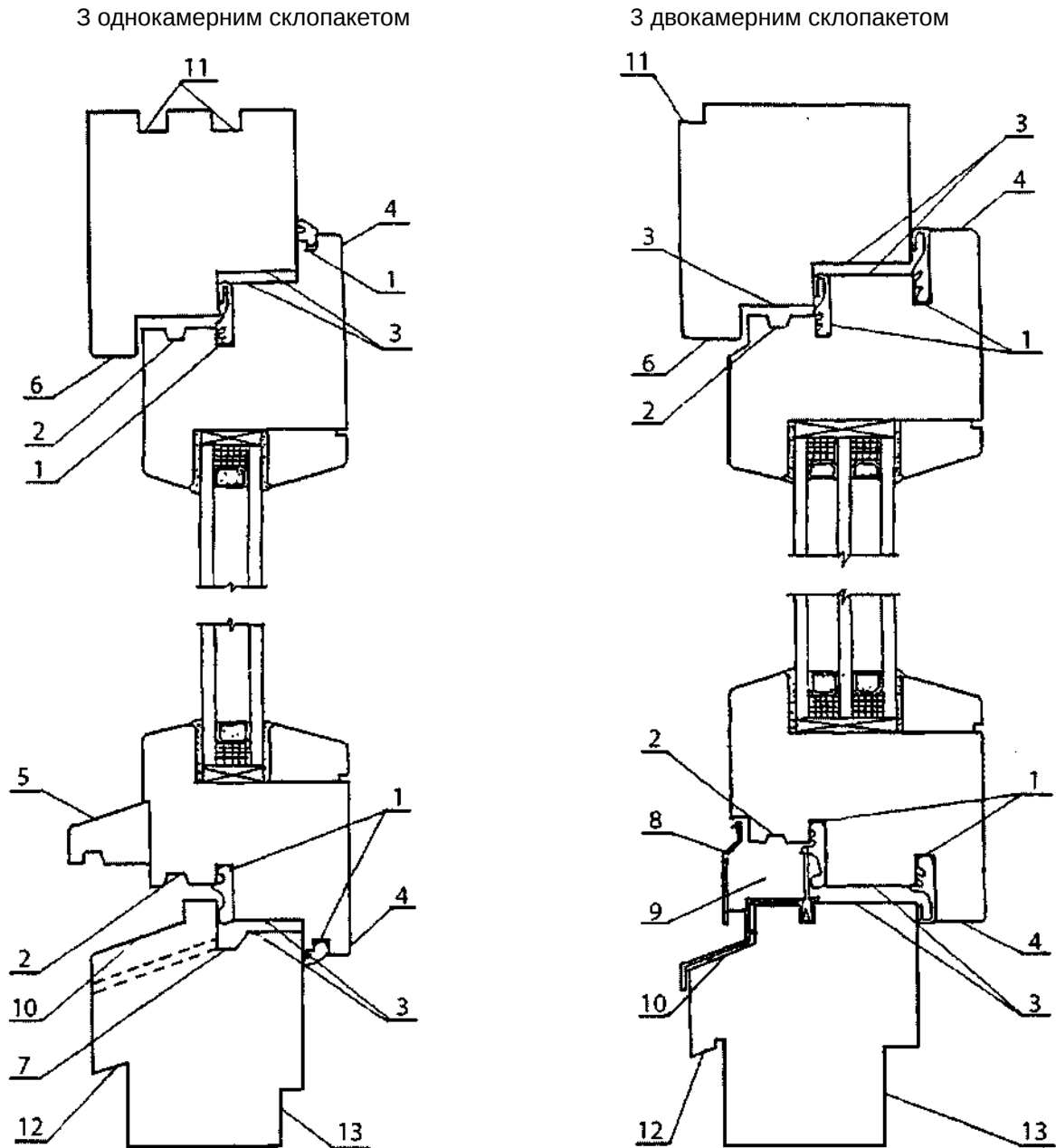
1 – паз під ущільнювальну прокладку; 2 – водовідвідна канавка; 3 – притульна частина; 4 – наплав стулки; 5 – відлив; 6 – наплав коробки; 7 – водовідвідний жолоб; 8 – дощозахисний профіль; 9 – водовідвідна камера; 10 – похил для відведення води; 11 – пази під з'єднувальні шпонки; 12 – чверть під злив; 13 – чверть під підвіконну дошку
