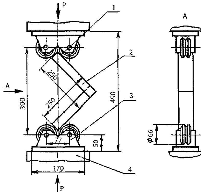
1 – точка прикладення навантаження; 2 – зразок; 3 – підпора; 4 – опора
